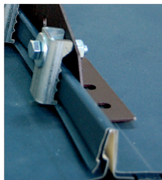
Кронштейн на Кликфальц® Pro (без затяжки)
