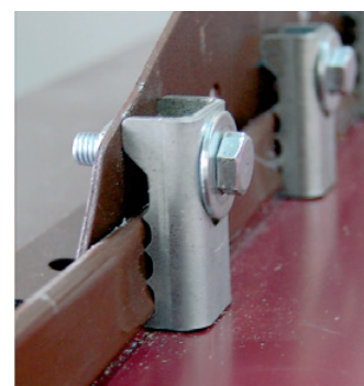
Кронштейн на Кликфальц® (с затяжкой)
